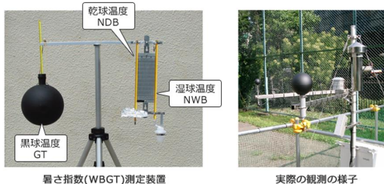
暑さ指数(WBGT)測定装置
